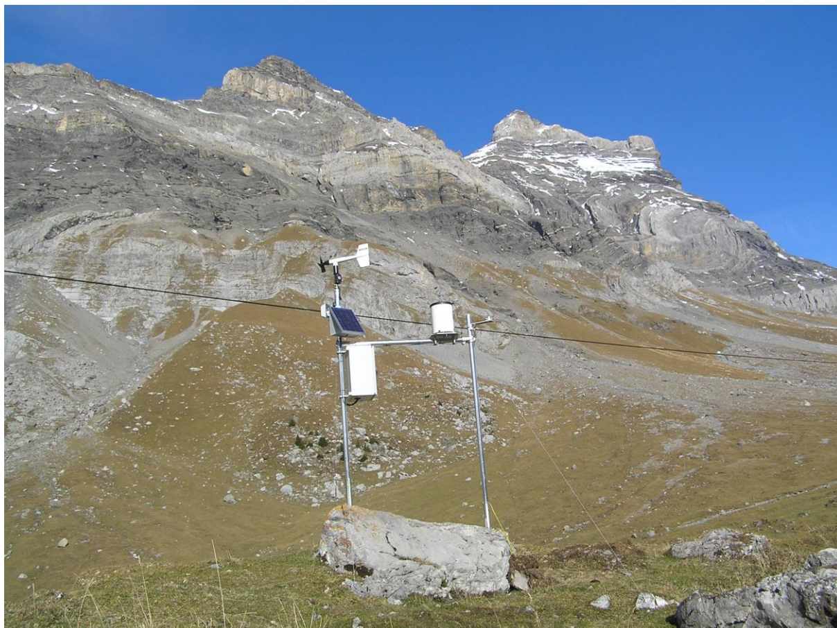
Figure 5 : Station météorologique d'Anzeindaz (1876 m/mer), au pied des Diablerets
